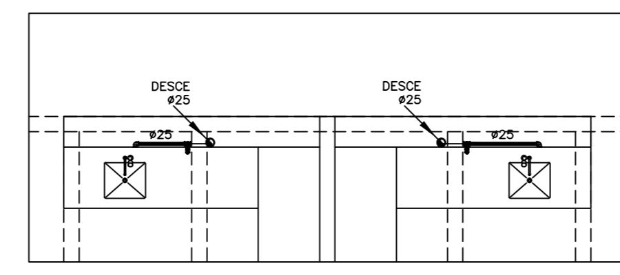
DETALHE-01 ESCALA 1:50
