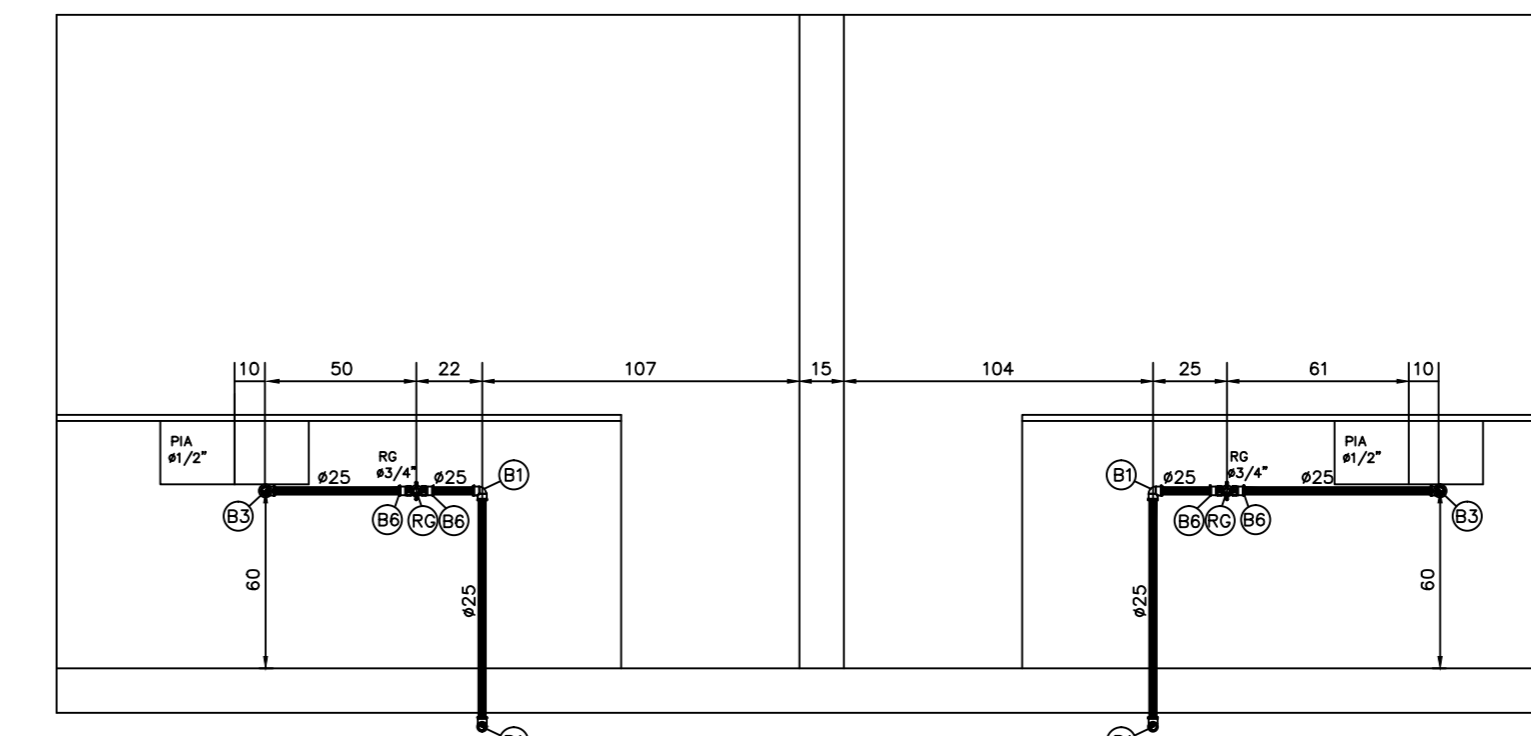
VISTA-1 ESCALA 1:25
